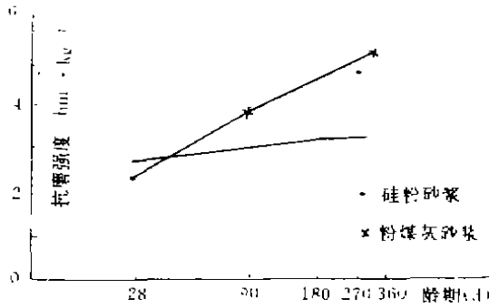
图2 天然河沙水泥砂浆的抗磨强度与龄期关系
