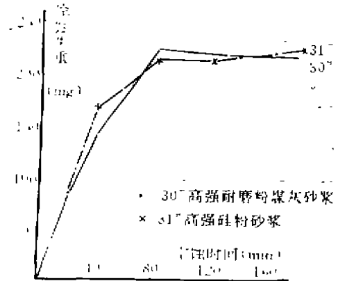
图5 砂浆空蚀失重随空蚀时间变化曲线
