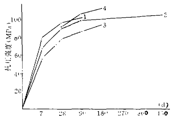
图1 粉煤灰砂浆(混凝土)随龄期变化曲线 注:1 粉煤灰铁矿石(混凝土);2 粉煤灰砂浆;3 粉煤灰混凝土;4 刘家峡现场试验,粉煤灰高强砂浆。
