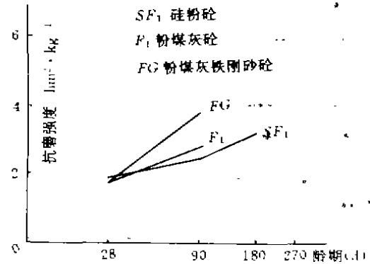
图4 几种混凝土抗磨强度与龄期关系
